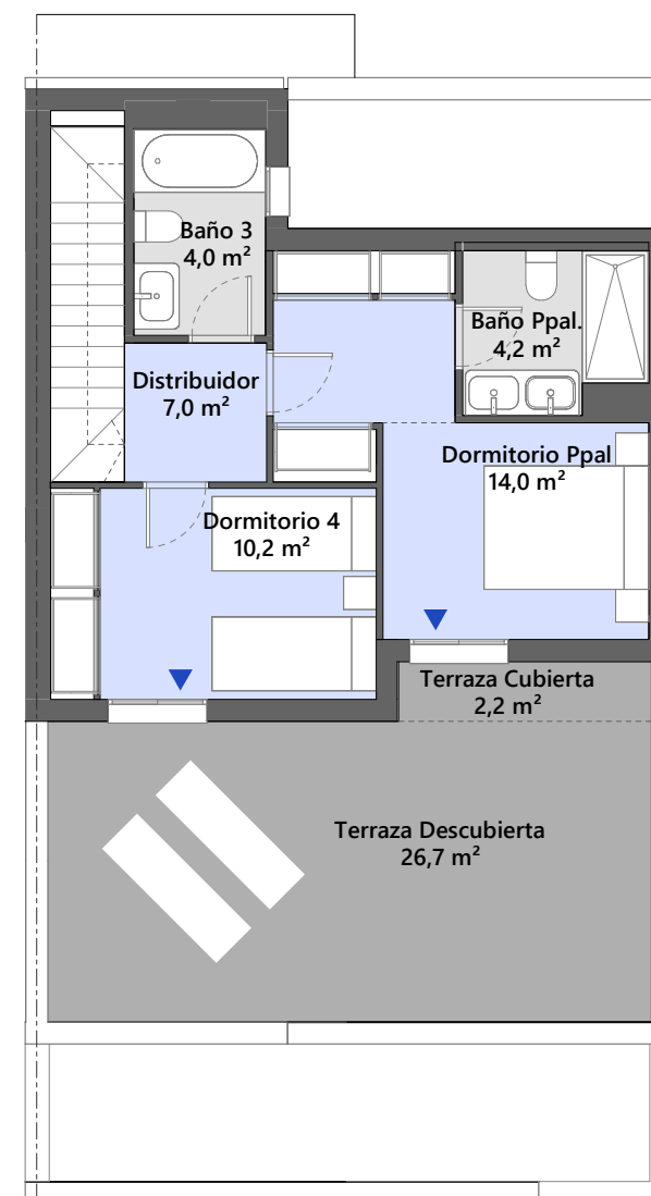
PLANTA PRIMERA
