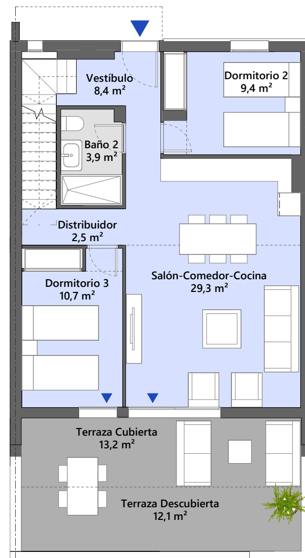
PLANTA BAJA
